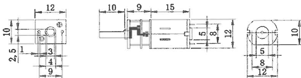
图 2 电动机尺寸参数（单位：mm）
